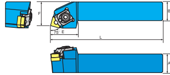
外徑車刀架 Tool holder
