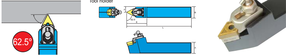
外徑車刀架 Tool holder
