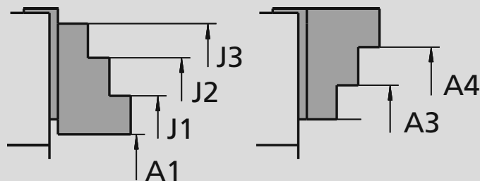
двухступенчатые накладные кулачки
