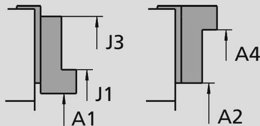
одноступенчатые накладные кулачки*
