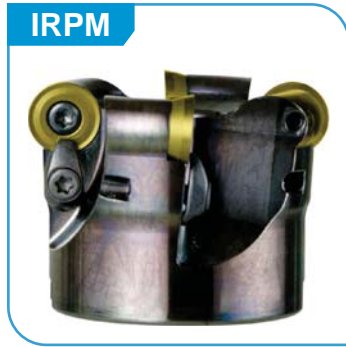
Radius Milling R角加工
